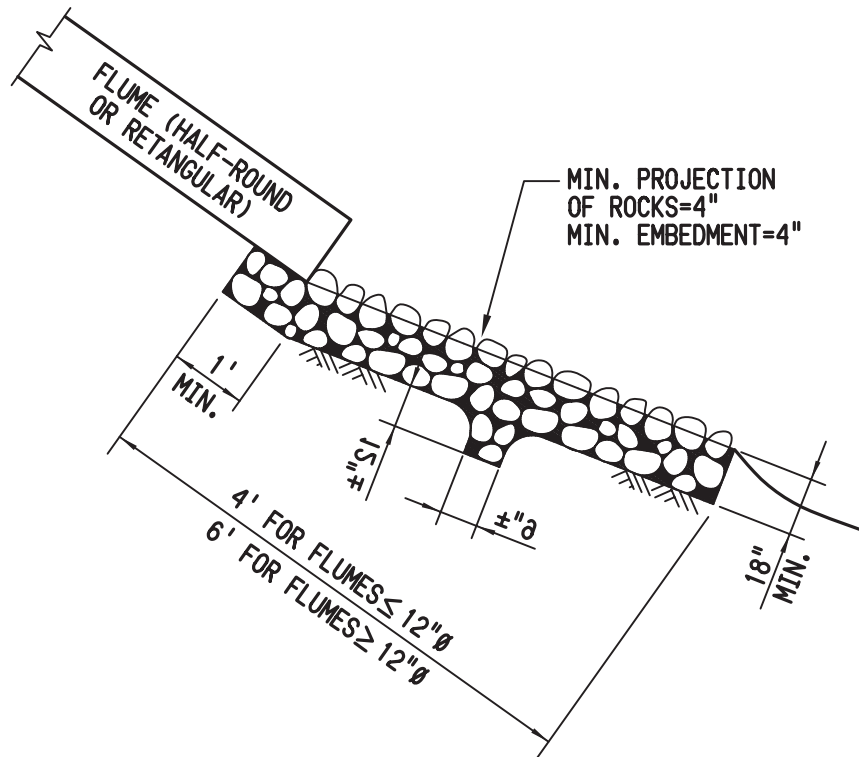
ELEVATION
